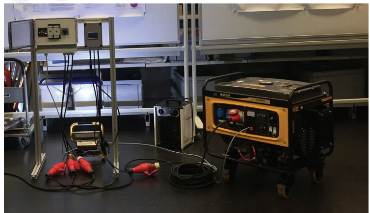
Unser Notstromaggregat auf Methanolbasis im Praxis-Test bei verschiedenen Blackouts
