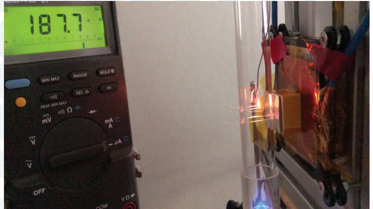
Messungen der vier Glasfasern und der Photovoltaik-Zelle an einem der Messstände der Econimo-Drive AG
